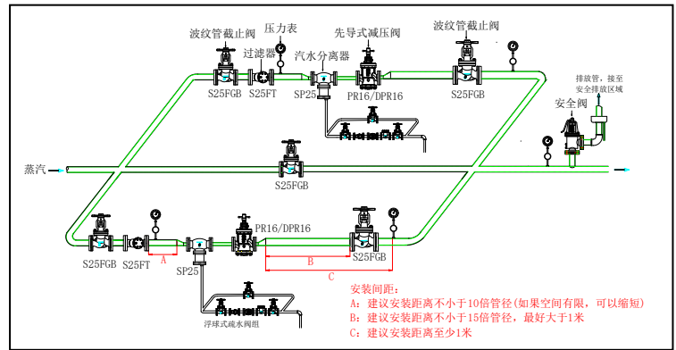
并联减压站示意图:
