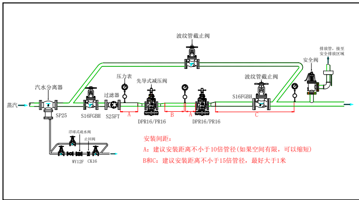
串联减压站示意图:
