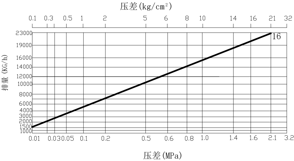
LFT45F (DN40~DN50) 排量表
