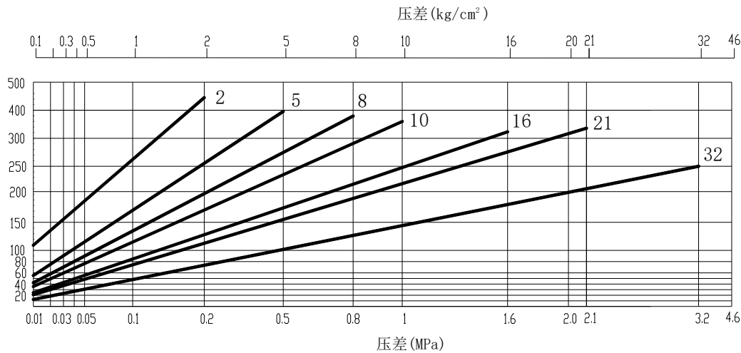
WY42S、WY42SU（DN15~DN25） 排量表
