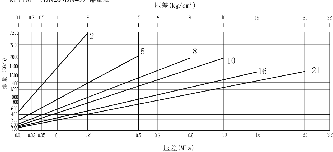
RFT18F（DN20~DN40）排量表
