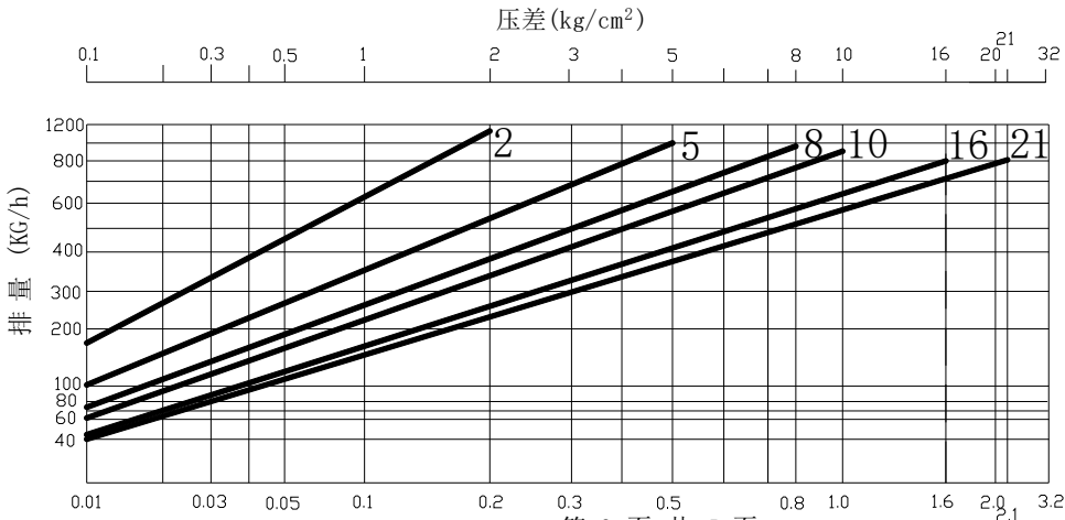
2. WY80FB 排量表
